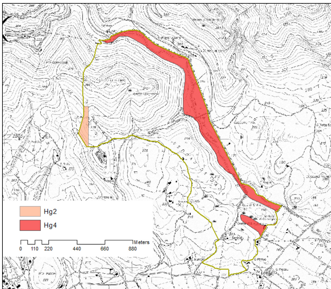
Figura 3. Stralcio del PAI in adeguamento. Sono rappresentate le diverse classi di pericolosità geomorfologica presenti all'interno dei limiti del SIC ITB042251 – "Corongiu de Mari"
