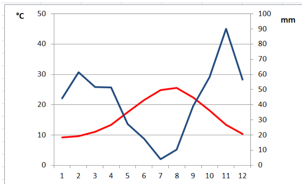
Figura 1. Diagramma termo-pluviometrico relativo alla stazione meteorologica di Decimomannu nel cinquantennio 1961-2010. La curva rossa indica le temperature, quella blu le precipitazioni.
