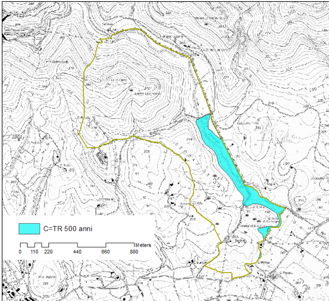
Figura 4. Stralcio del PSFF. Rappresentazione delle fasce fluviali identificate dal PSFF all'interno dei limiti del SIC ITB042251 – "Corongiu de Mari"
